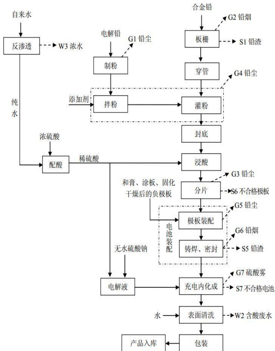
图 3-3 牵引性蓄电池生产工艺流程图
