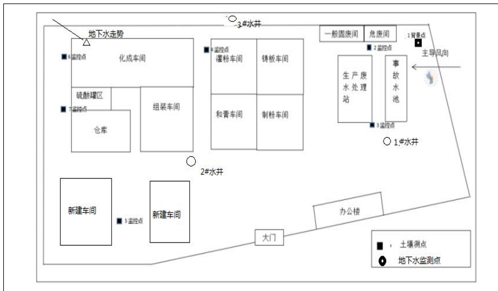
图 3-1 厂区平面图
